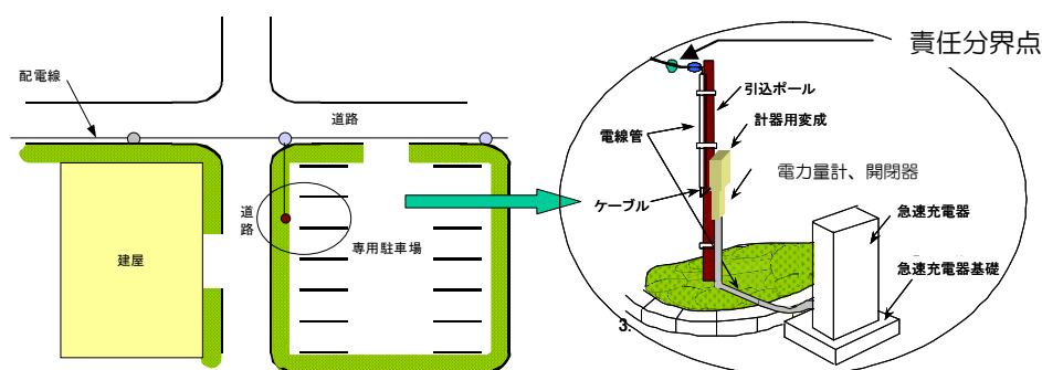
図3-2-1 急速充電器の低圧供給の一例
